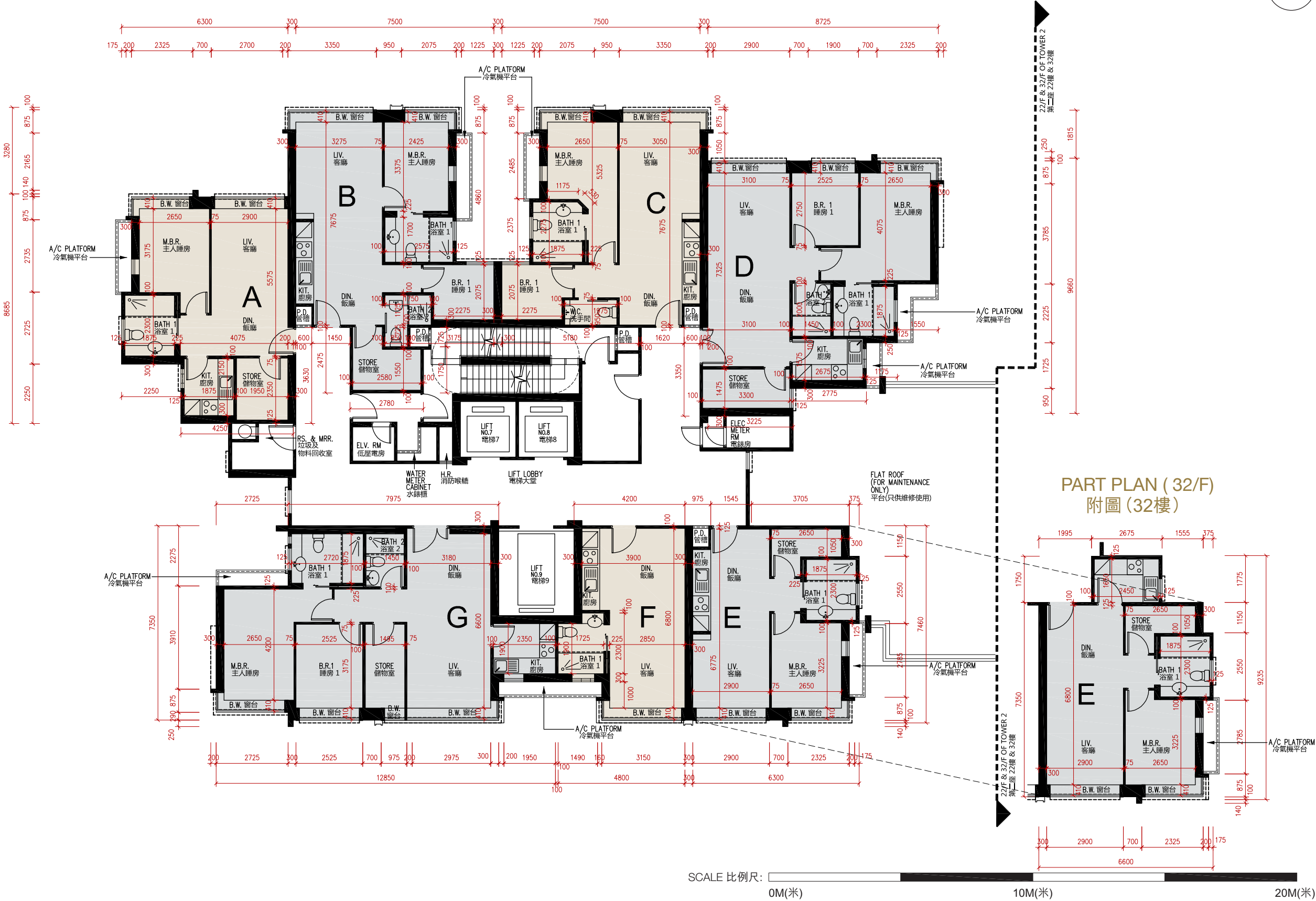
22/F AND 32/F OF TOWER 3 FLOOR PLAN 第三座22樓及32樓平面圖
