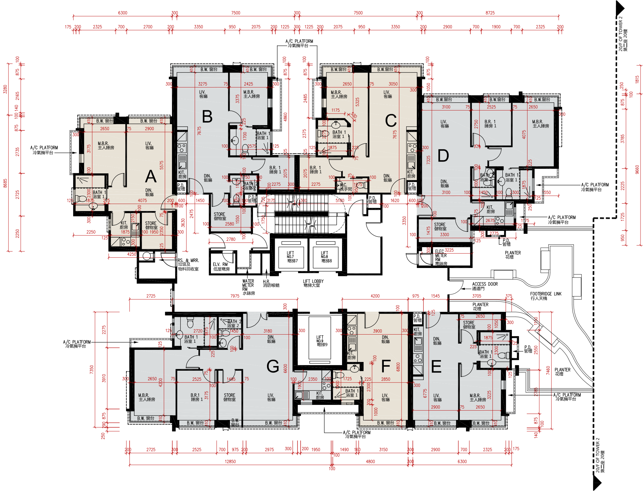
20/F OF TOWER 3 FLOOR PLAN 第三座20樓平面圖
