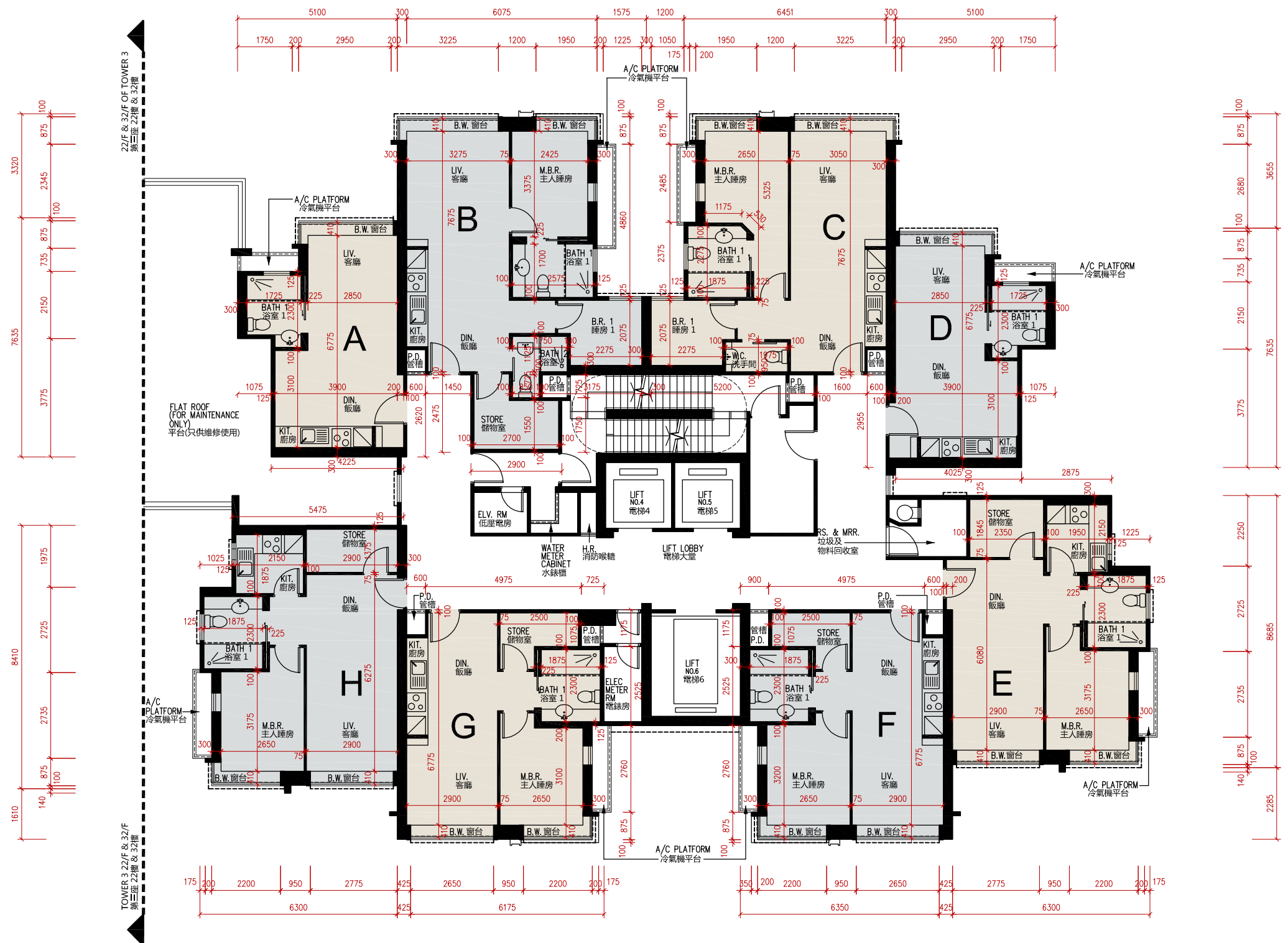
22/F AND 32/F OF TOWER 2 FLOOR PLAN 第二座22樓及32樓平面圖
