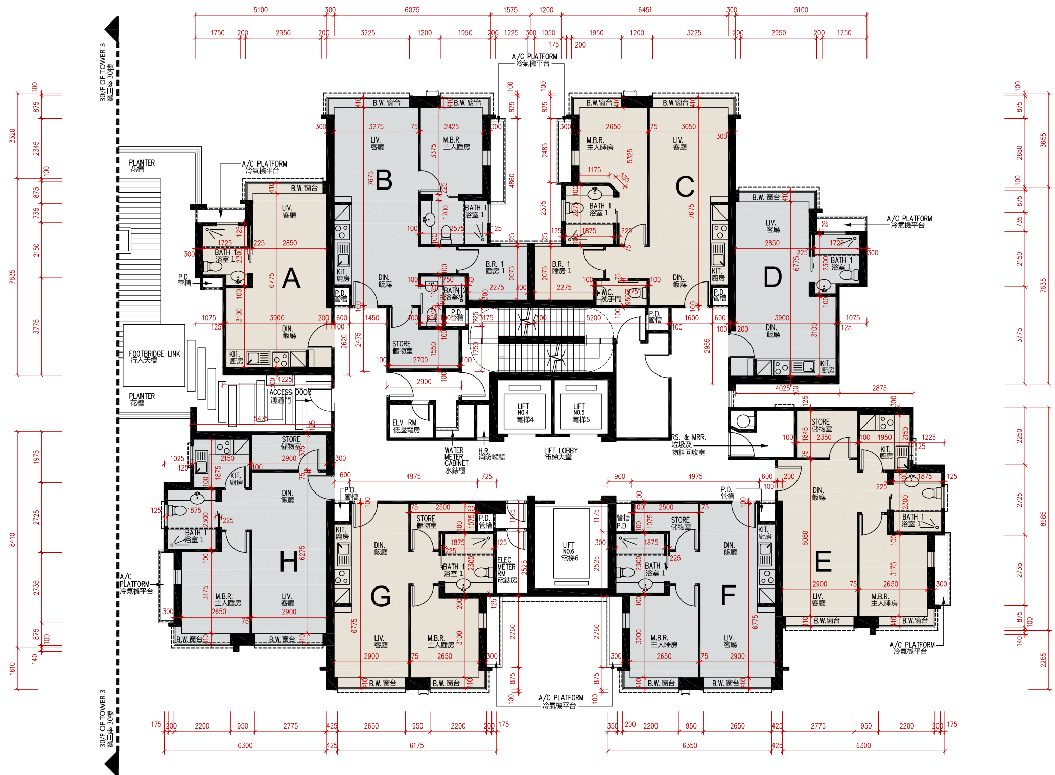
30/F OF TOWER 2 FLOOR PLAN 第二座30樓平面圖
