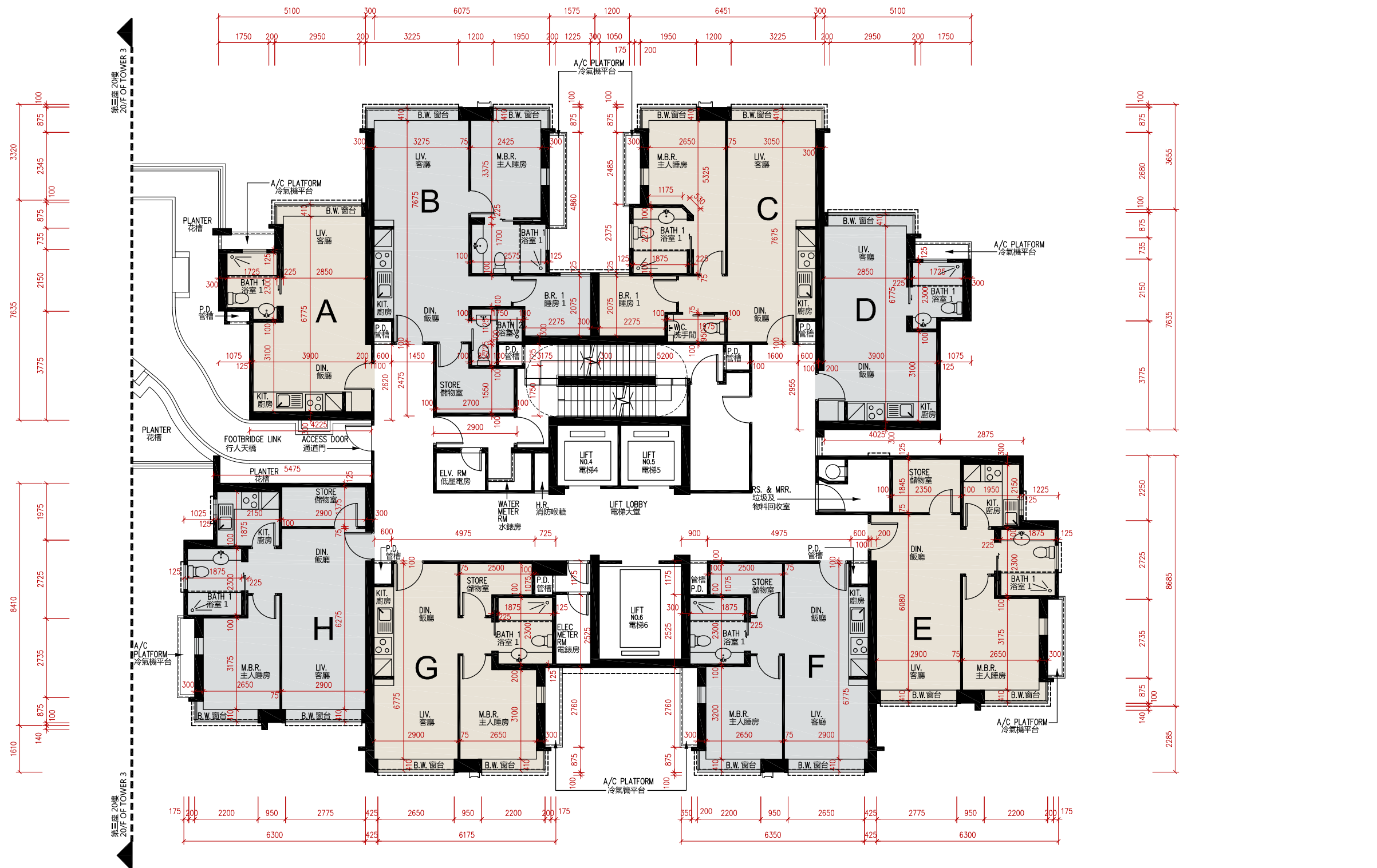
20/F OF TOWER 2 FLOOR PLAN 第二座20樓平面圖
