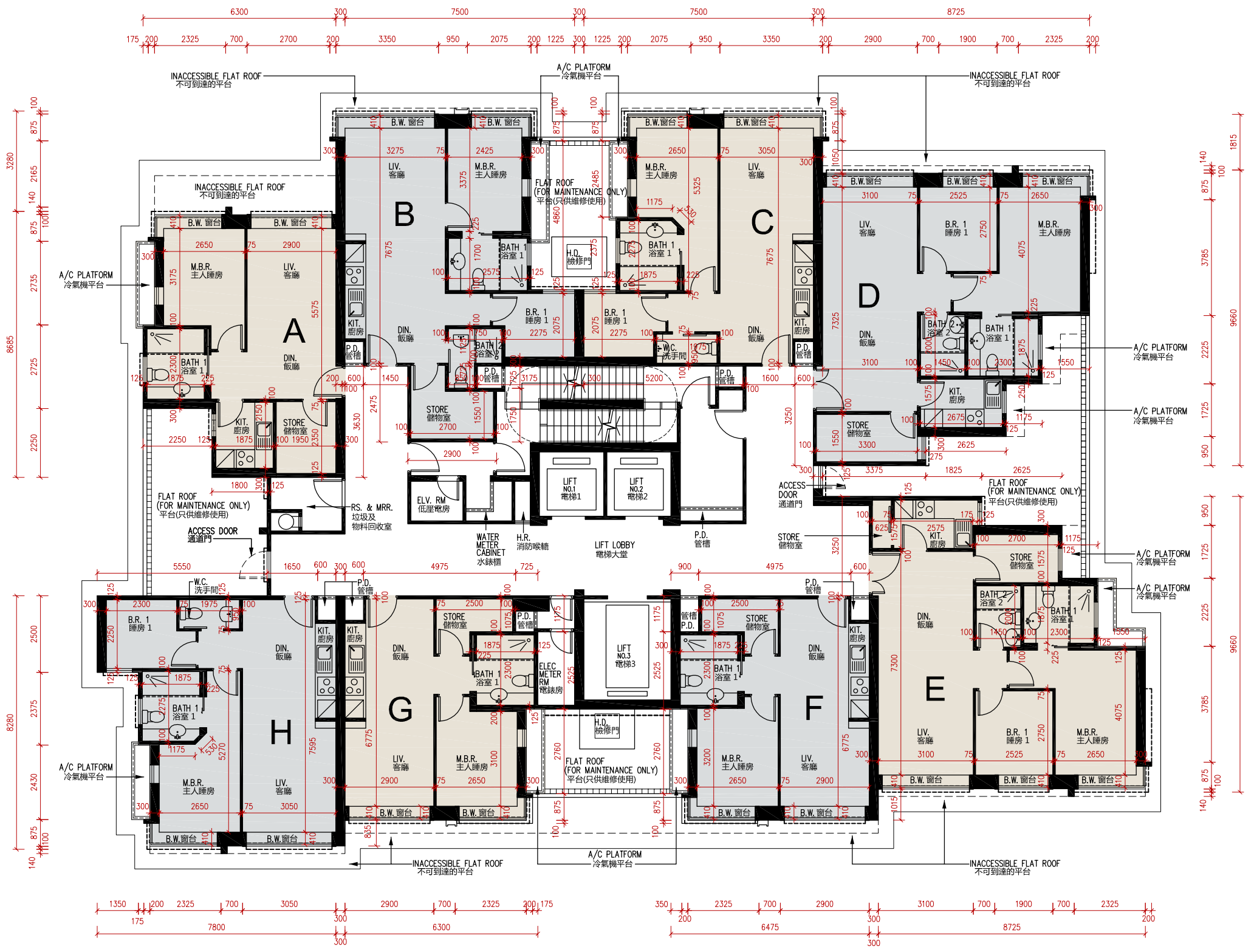
6/F OF TOWER 1 FLOOR PLAN 第一座6樓平面圖
